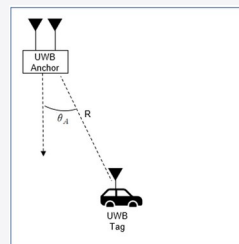
제안 · 1-Anchor AoA + DS-TWR
